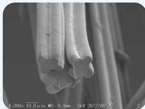
糸断面電子顕微鏡写真
